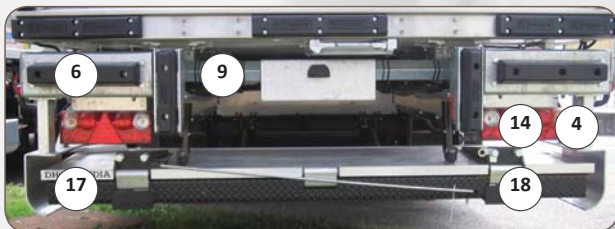
1.1 Module Arrière hayon avec butoir et avec protection latérale
