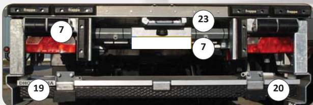
1.2 Module Arrière hayon avec protection (avant 2008)
